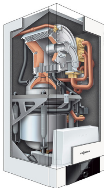
Ein Schnittbild einer Erdgas-Therme mit Stirling-Generator. Die elektrische Leistung wird mit 1 kW angegeben, die thermische mit 6 kW im Normalbetrieb und mit bis zu 20 kW bei Spitzenlast. [Grafik: Viessmann]
