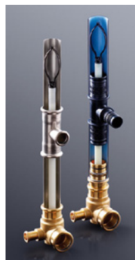
Ein flexibles Kunststoffrohr, welches in die Warmwasser-Steigleitung eingeschoben wird, fungiert als Zirkulationsleitung. [Bild: GEBERIT]
