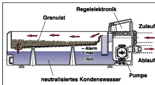
Schnitt durch eine Neutralisationsbox [Grafik: BUDERUS]
