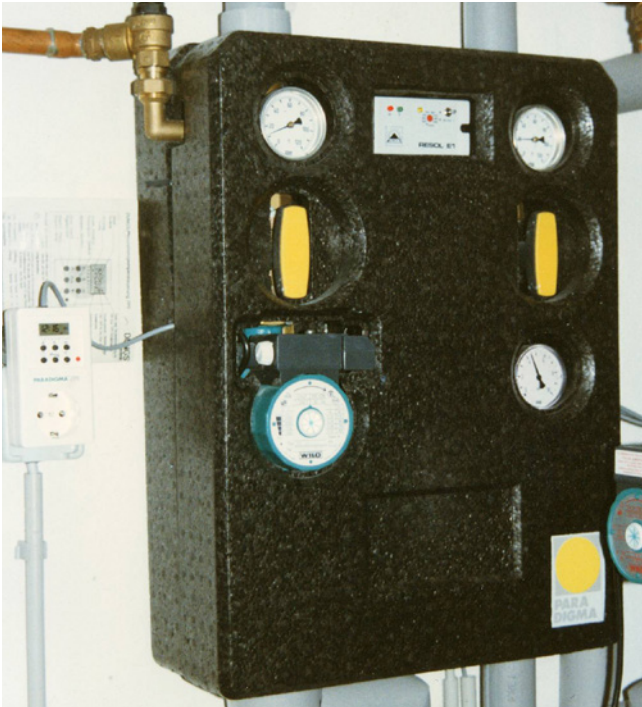
Solarstation: Pumpe, Thermometer, Manometer und Absperrventile sind zusammen in eine Dämmschale eingebaut.
