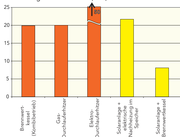
Primärenergiebedarf in kWh/(m 2 a)
