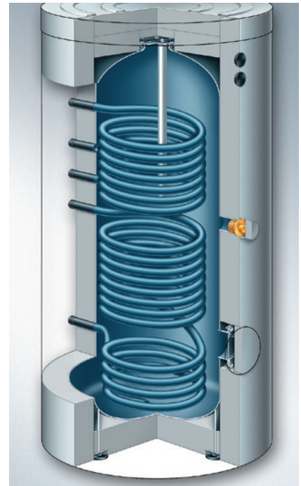
Schnittzeichnung eines Edelstahlspeichers: Unten der Wendel des solaren Wärmetauschers, oben der für die Nachheizung. Brauchwasser unter Leitungsdruck füllt den gesamten Speicher
