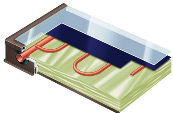
Schnittbild eines Kollektors:
