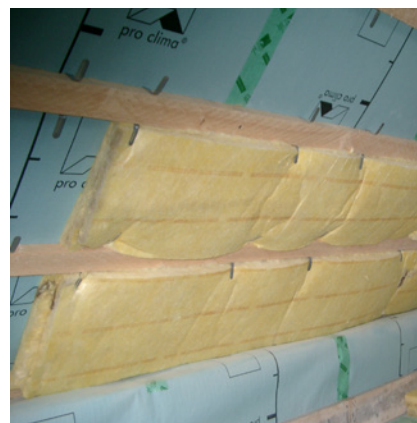
Untersparrendämmung 50 mm zwischen der Unterkonstruktion
