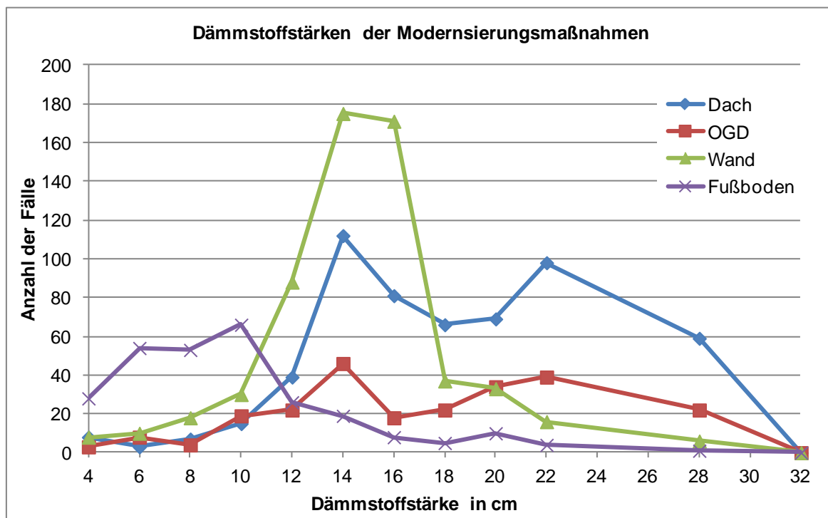
Abbildung 6 Energieeffizient Sanieren 2011: Dämmstoffstärken der durchgeführten Modernisierungsmaßnahmen (gesamte Stichprobe, tatsächliche Dämmstoffdicke ohne Berücksichtigung der Wärmeleitfähigkeit)
